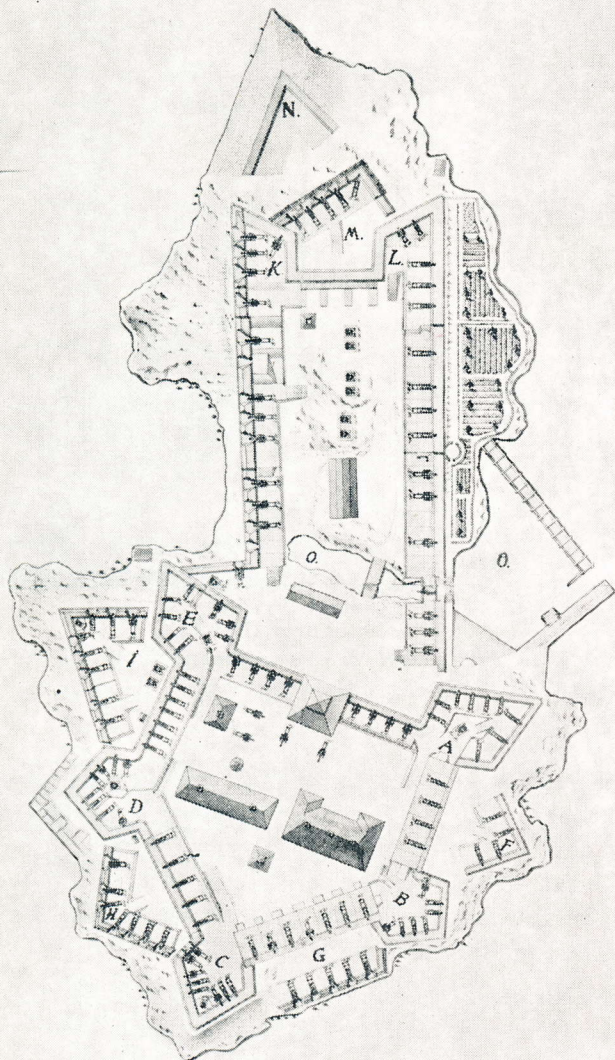
Plan av Nya Älvsborg 1790. Vid inre hamnen ligger sjukhuset. På inre gården corps-degarde, kommandantshus och stenkasern. A bastionen Nordstjernen, B Delfinen, C Havsfrun, D Valfiscen, E Hummern, F ravelinen Prins Fredrik, G Stenbatteriet, H ravelinen Rosenlund, I Vedgården, K Västra hornet, L Östra hornet, M Smedjebatteriet, N Stenglacien, O yttre hamnen och därovan kommandantens trädgård. Kungl. Krigsarkivet.
